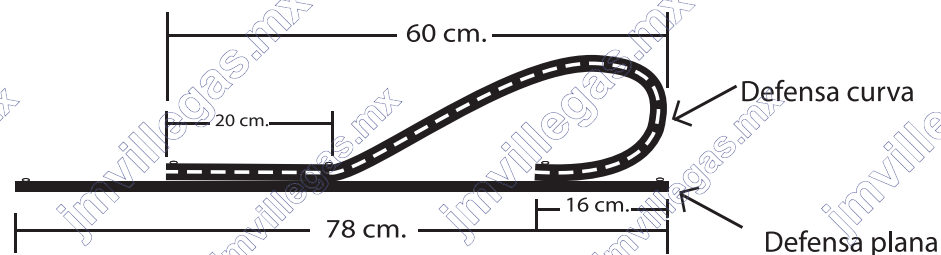
Defensas plana y curva (detalle de perfil)
